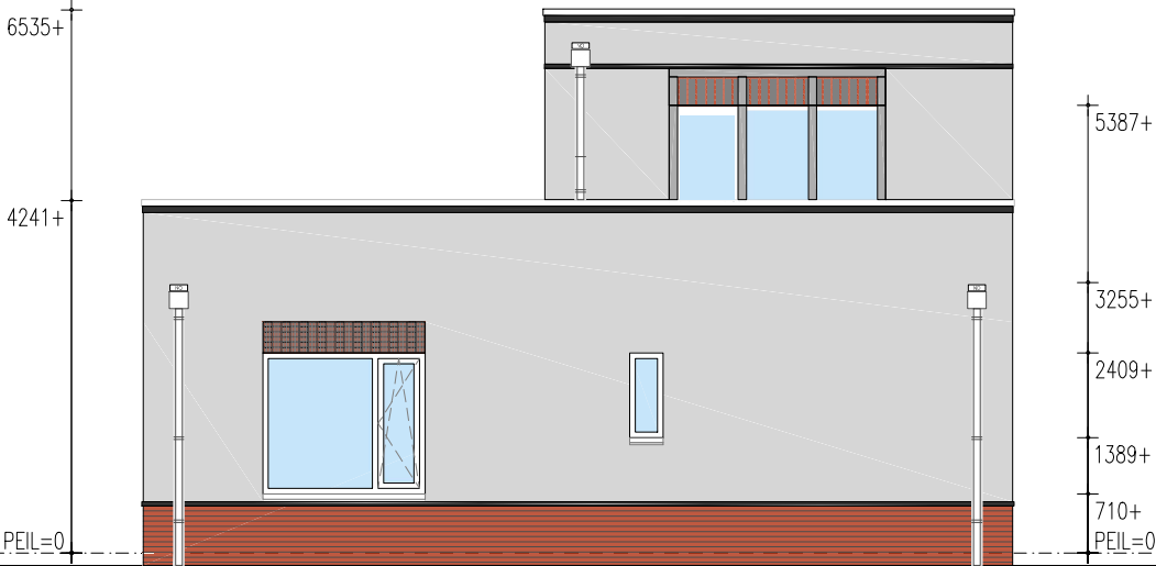
BNR. 17 Linker zijgevel
