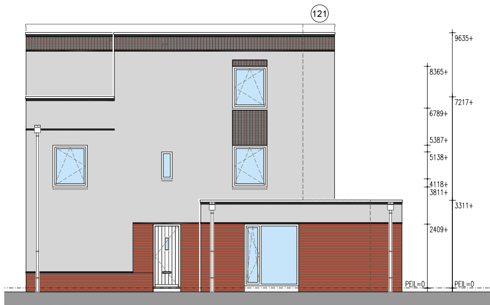
Rechter zijgevel
