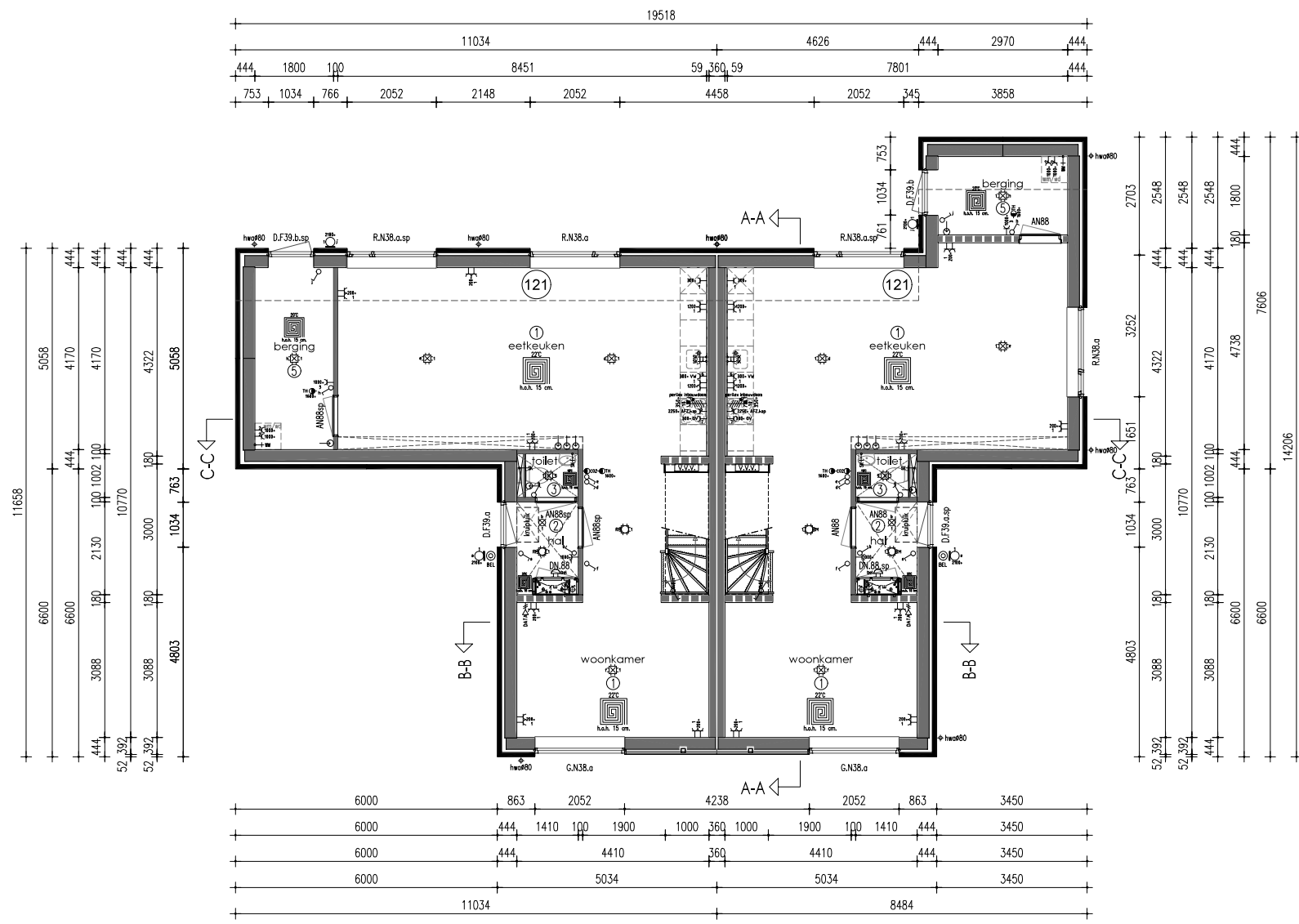
Begane grond
