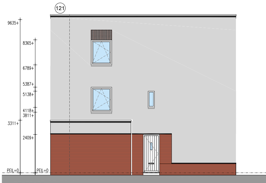
Linker zijgevel
