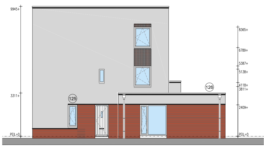
Rechter zijgevel
