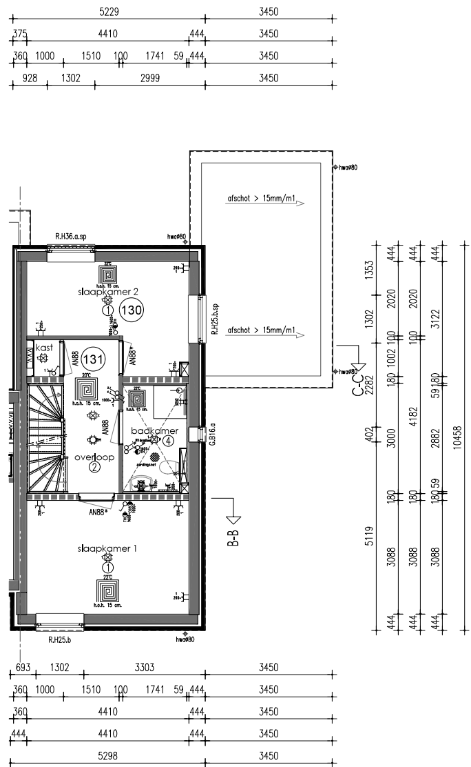
1e Verdieping
