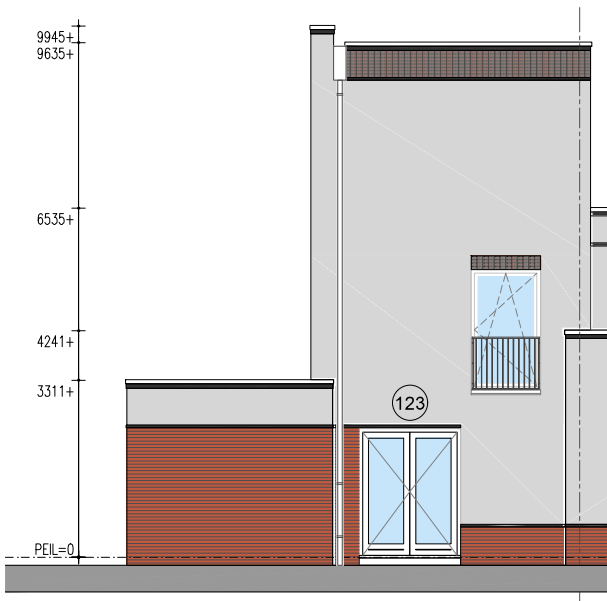
Achtergevel
