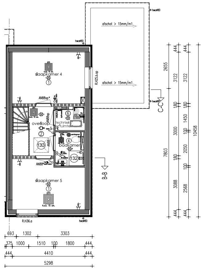
2e Verdieping
