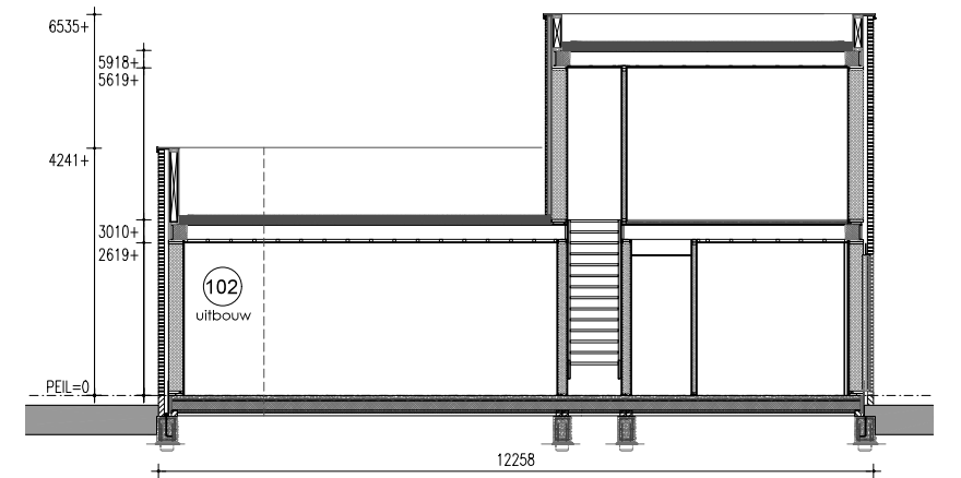
PRINCIPE DOORSNEDE A-A
