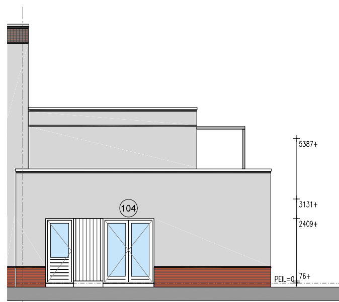
Achtergevel
