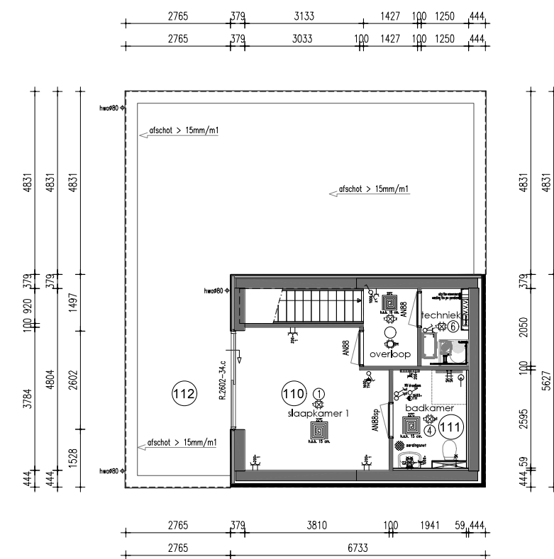
BNR. 17 1e Verdieping
