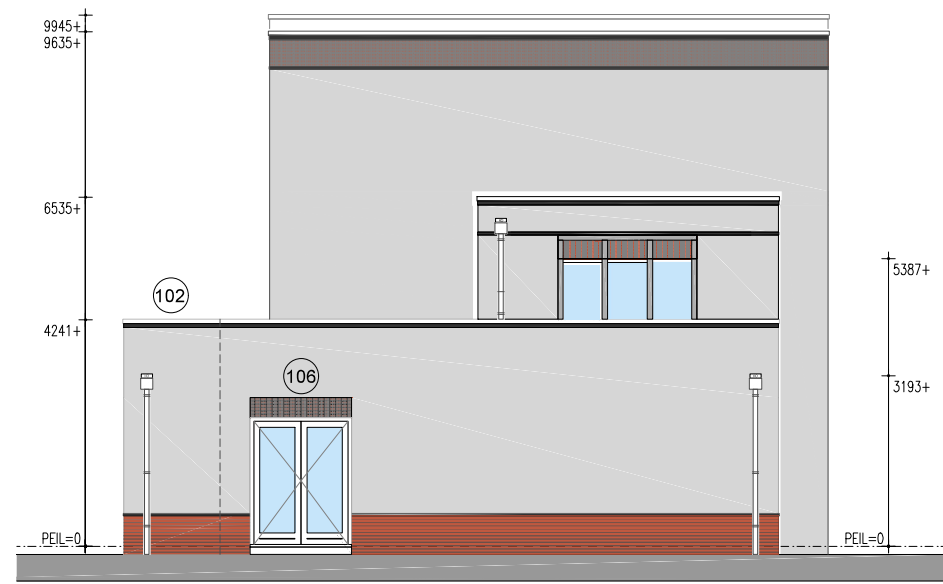
Linker zijgevel
