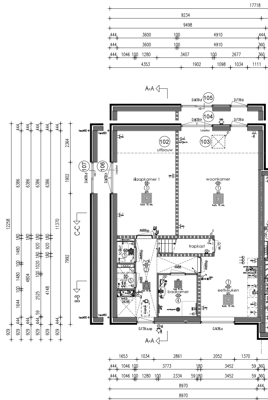
Begane grond
