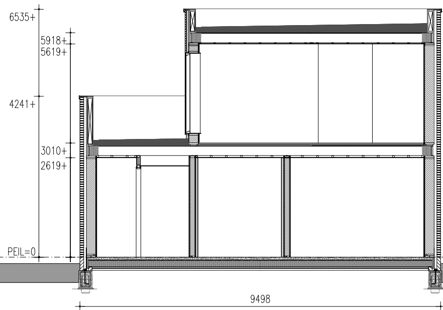
BNR. 05 PRINCIPE DOORSNEDE B-B
