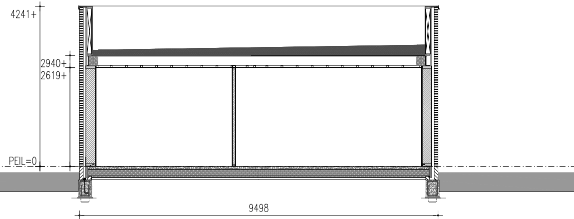
BNR. 05 PRINCIPE DOORSNEDE C-C
