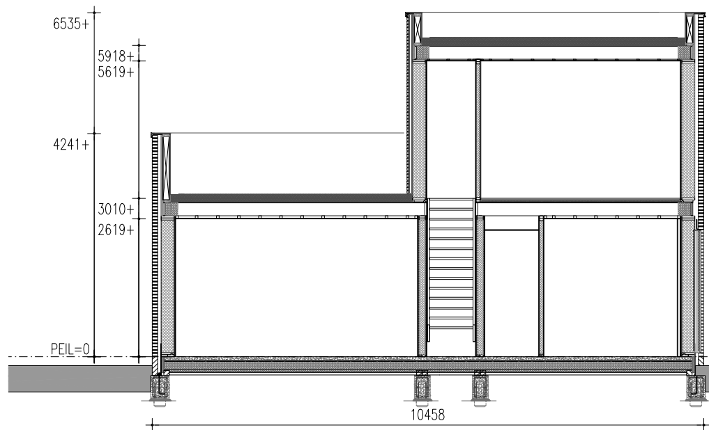
BNR. 05 PRINCIPE DOORSNEDE A-A
